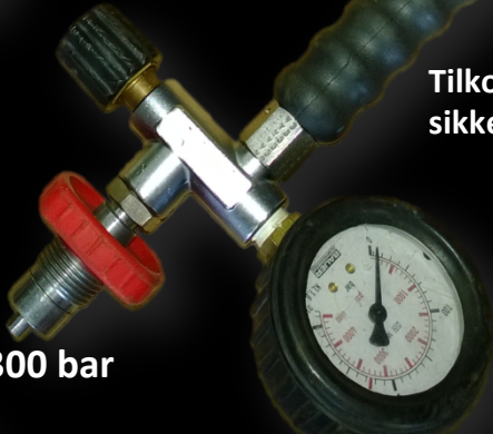
Tilkoblet 300 bar sikkerhetsventil med 200 bar fyllenippel
